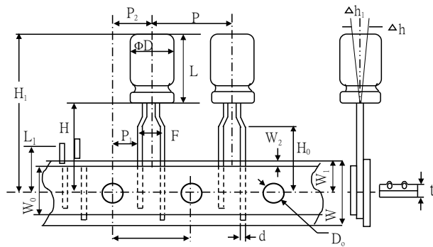
Fig.3(Φ5-Φ8)
