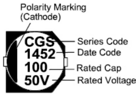
Chip Type Fig.1 ØD=6~10mm
